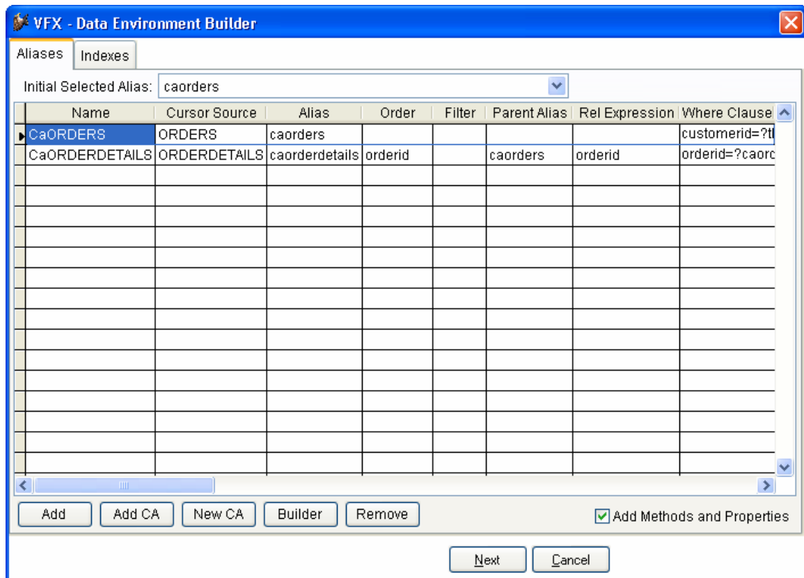
Relationen und Where-Klauseln im VFX – Data Environment Builder
